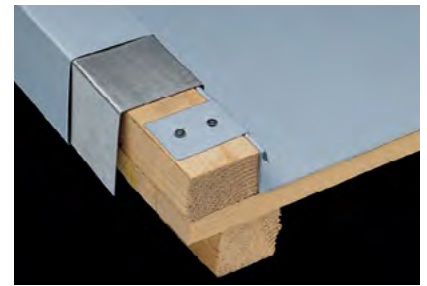
Гребень с брусом
