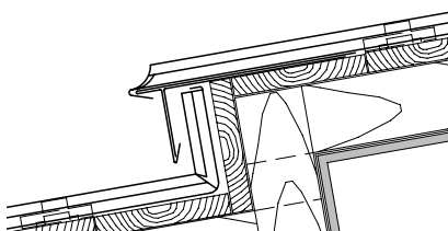
Фальц конвертом на перепадах
