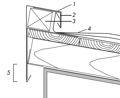
Конек односкатной кровли с брусом кровли
