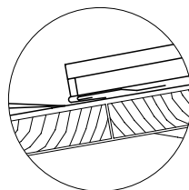
Оптимизация узла: дополнительная планка
