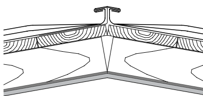
Гребень с профилем
