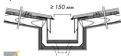
Внутренний желоб с клееным страховочным желобом
