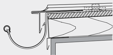
Свес кровли – неправильное исполнение узла
