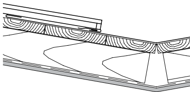
Ендова с простым и дополнительным фальцем
