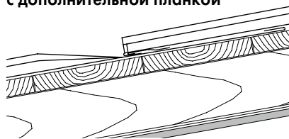
Поперечный шов – простой фальц с дополнительной планкой
