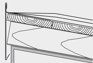
Конек односкатной кровли без деформационной зоны, небольшой торцевой фальц
