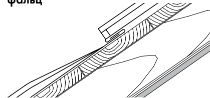
Поперечный шов, как простой фальц
