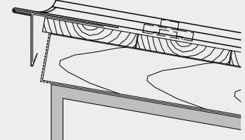
Конек односкатной выполнен как карниз
