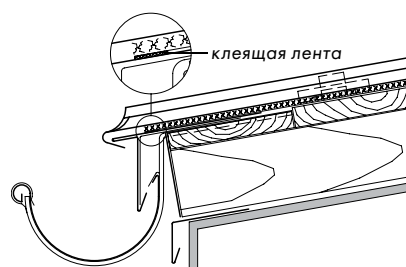
Окончание свеса кровли с ОДМ
