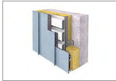
Вентилируемая подконструкция 2 из металла
