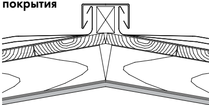
Гребень с брусом и профилем покрытия
