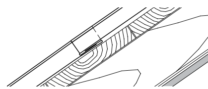
Фальц в фальц – поперечный шов для углового стоячего фальца
