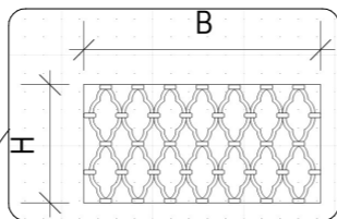
Фасад 1-3 (северный фасада)
